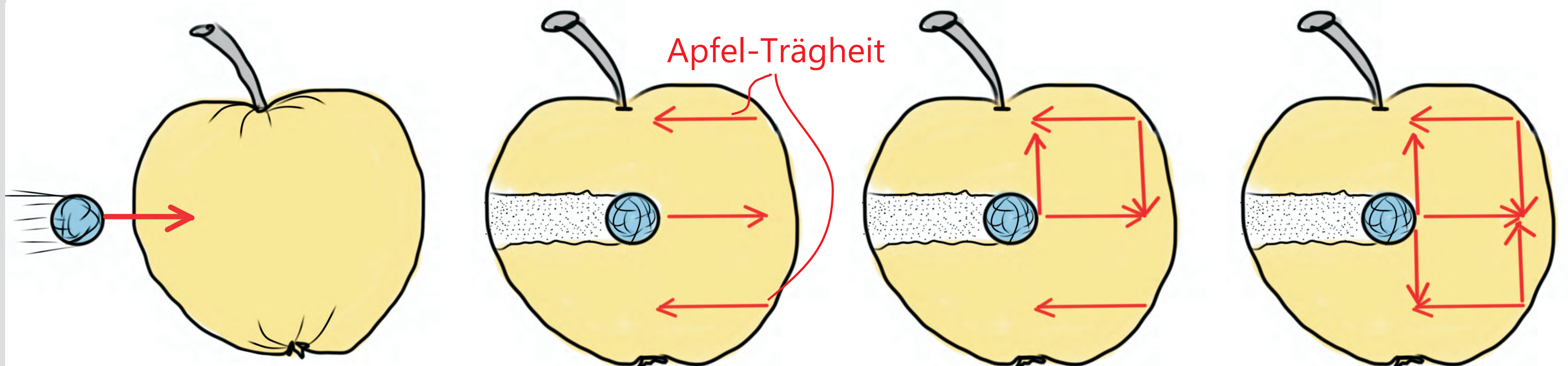
Stanzendes Schubversagen
